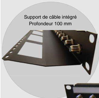
Panneau de brassage 1x16 F/F
